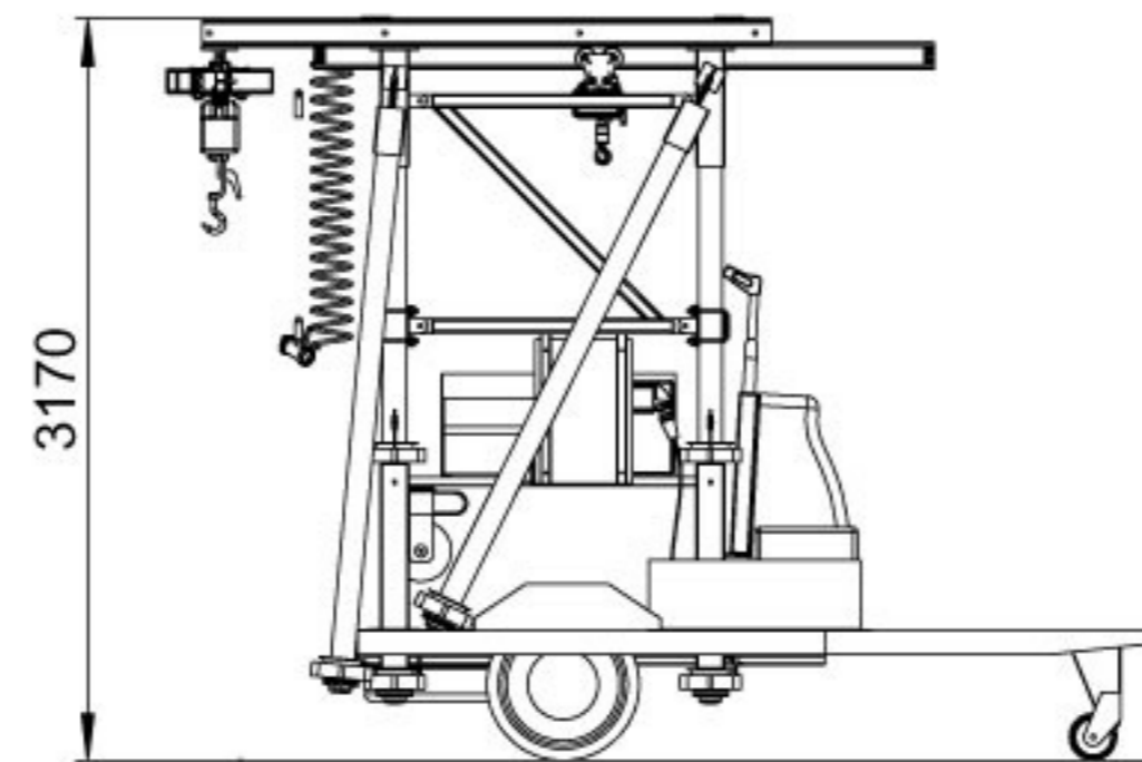
Transportstellung
