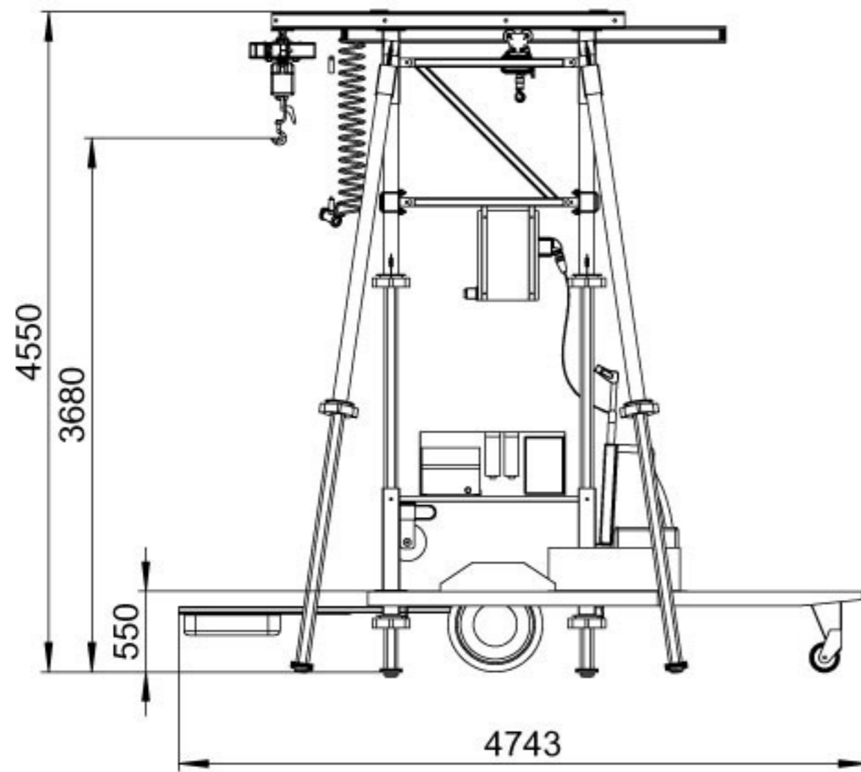
Arbeitsstellung
